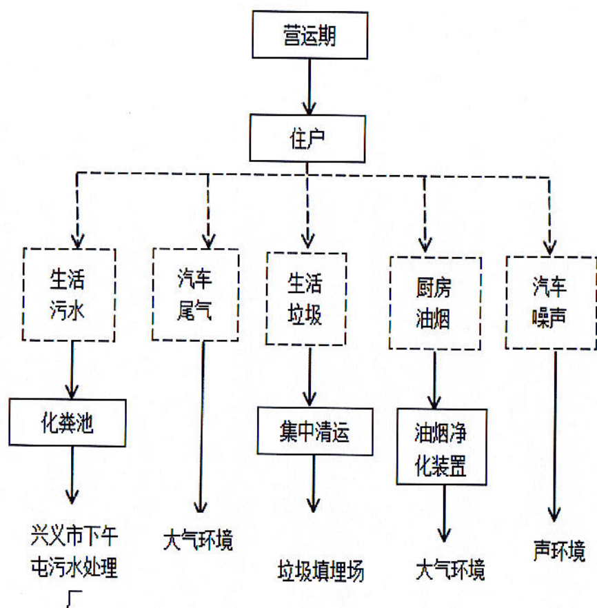
图 1 工艺流程及产污节点图
