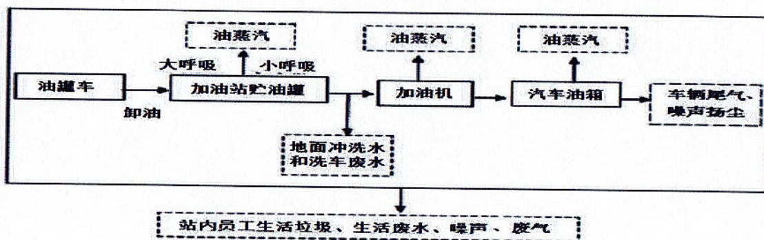
图 1 运营期工艺流程及产污节点图
