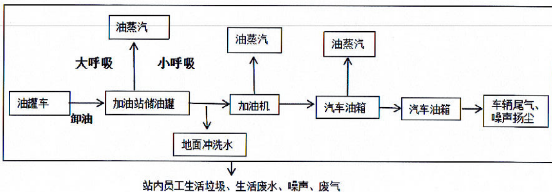
图 1 加油工艺流程和产污节点图
