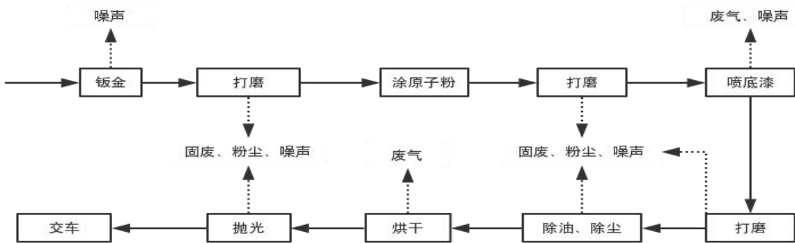
图 2-4 运营期喷漆工艺流程及产污节点
