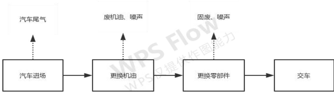
图 2-2 运营期保养工艺流程及产污节点
