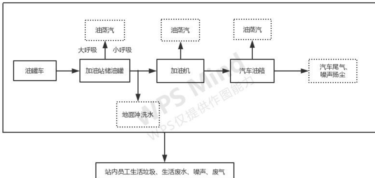
2-3加油工艺流程和产污节点图
