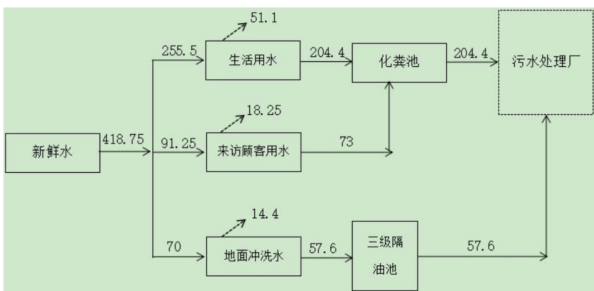
2-2 项目水平衡图 (t/a)
