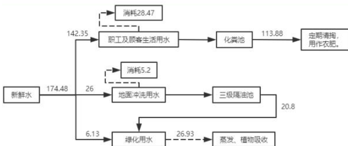
2-2 项目水平衡图 (t/a)
