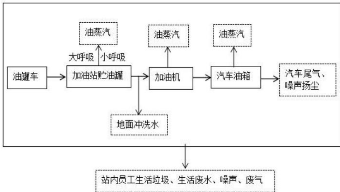
2-3加油工艺流程和产污节点图
